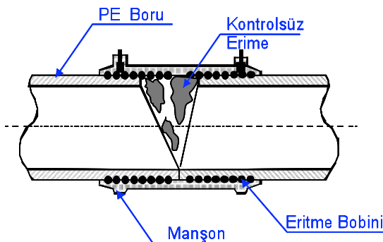
Düzgün kesilmeyen boru uçlarının kaynağa olumsuz etkisi
