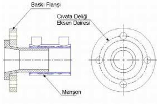
Tipik flanş bağlantı detayı
